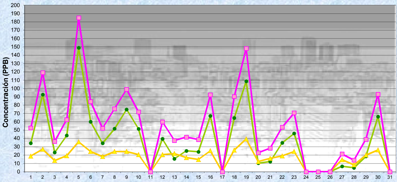
AGOSTO 2016 Concentración promedios de 8 hs de 8 a 16 Hs
