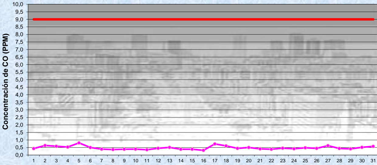
OCTUBRE 2017 Concentración de CO- promedios de 8 hs
