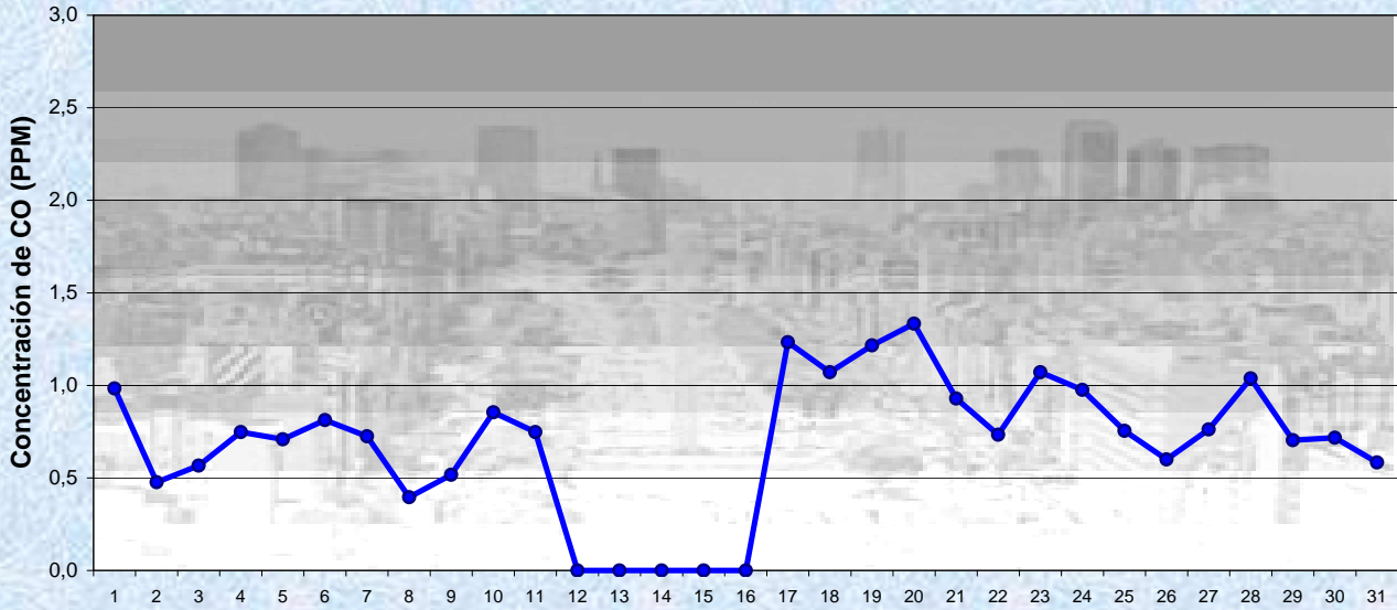
JULIO 2012 Concentración diaria de CO ● Promedio 24 Hs
