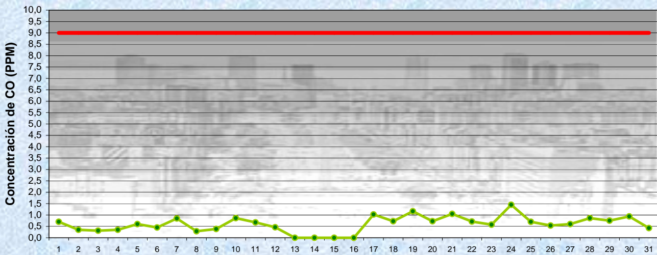
JULIO 2012 Concentración de CO- promedios de 8 hs ● CO de 0 a 8 hs — Valor límite admisible: 9 PPM en 8 Hs (Ley 1356-GCBA/ NAAQS-EPA)
