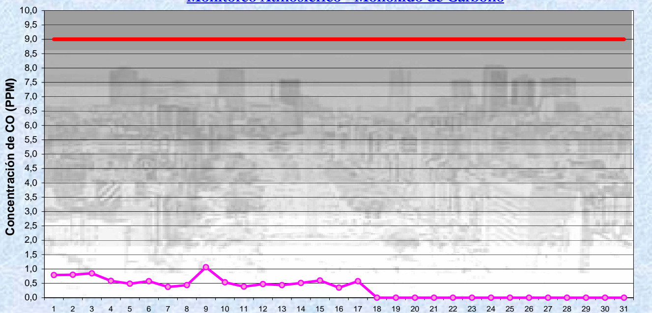
DICIEMBRE 2008 Concentración de CO- promedios de 8 hs
