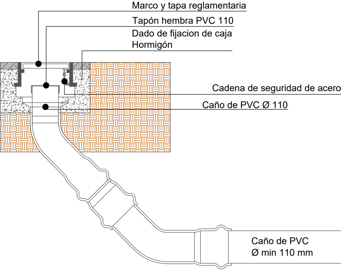
CORTE 1:10
