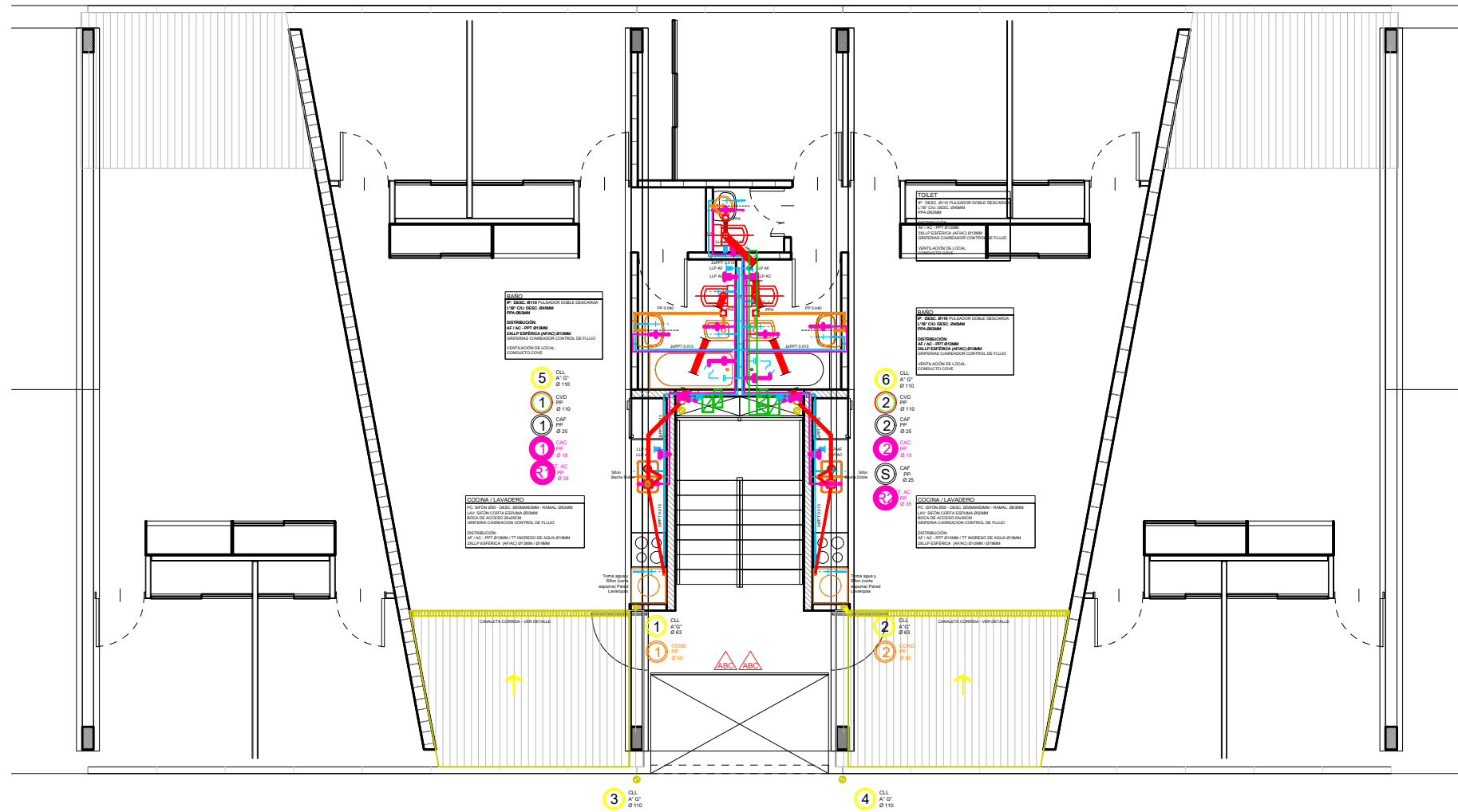
PLANTA TIPO
