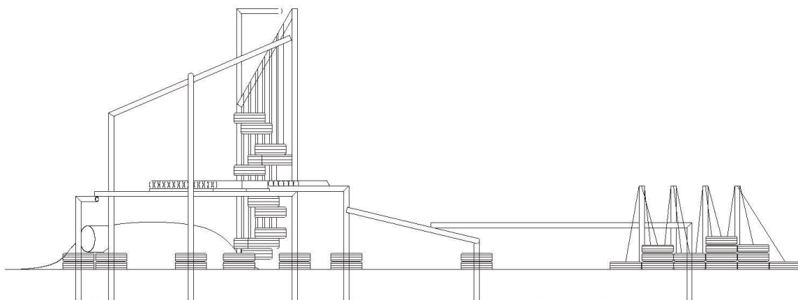
JUEGO DE PLAZA: CASA DE LOS CHINGOLITOS PLANTA + VISTA ESC. 1:25
