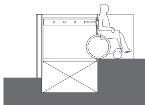
corte horizontal
