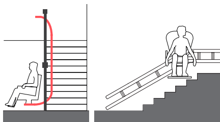
corte transversal
