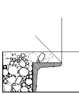
DETALLE E
