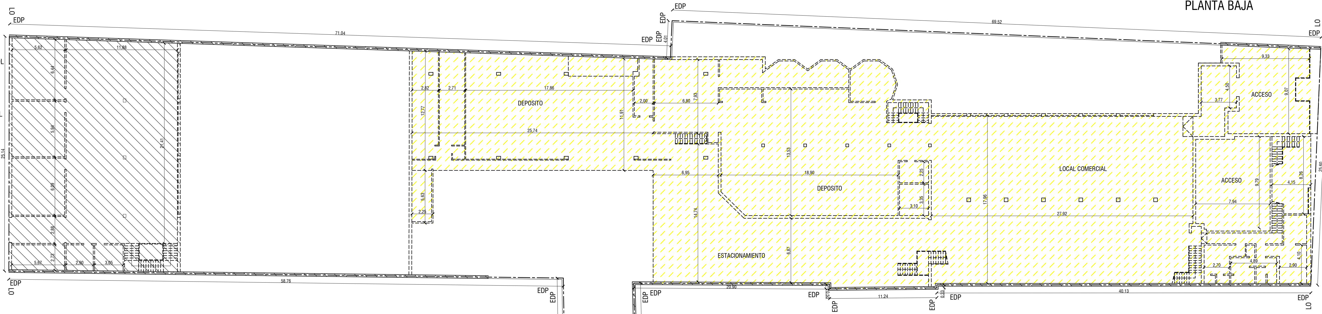
PLANTA BAJA
