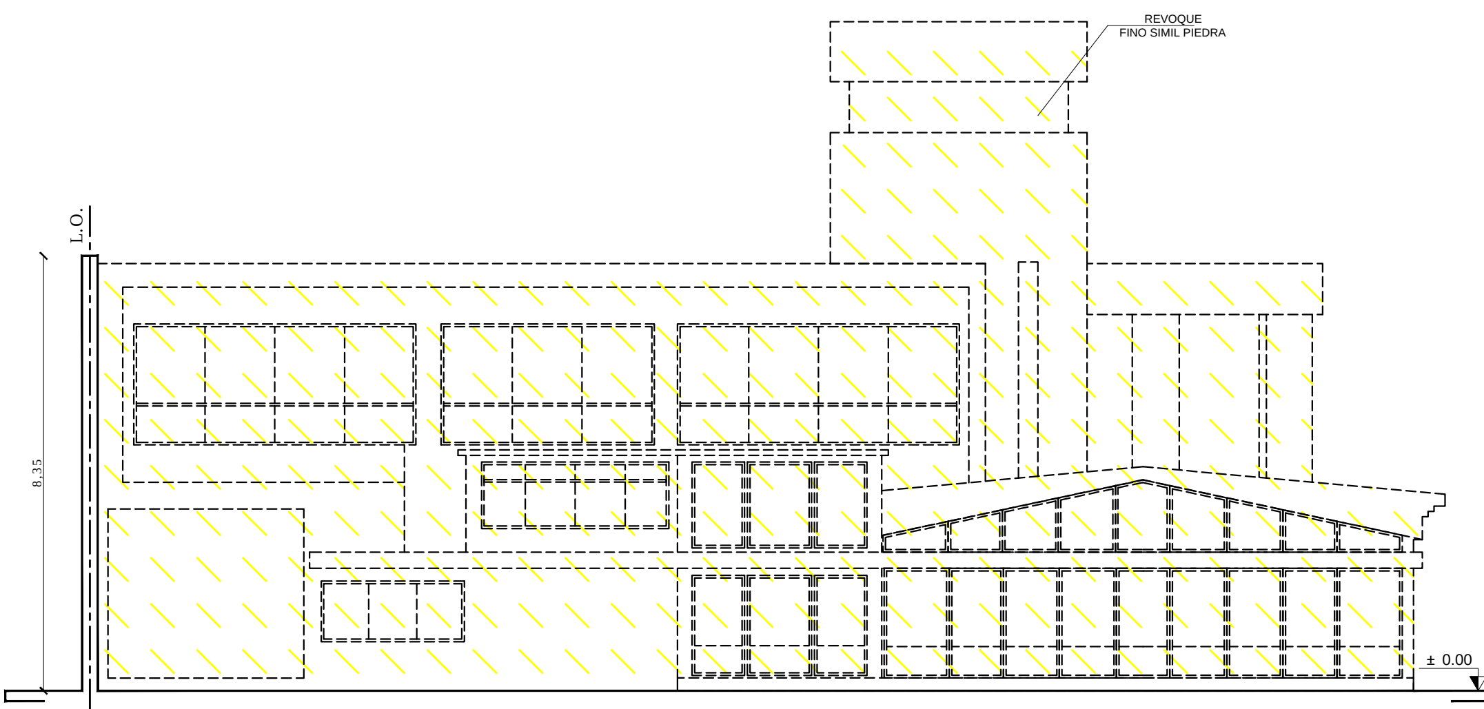
FACHADA
