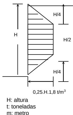
Diagrama de presiones horizontales:
